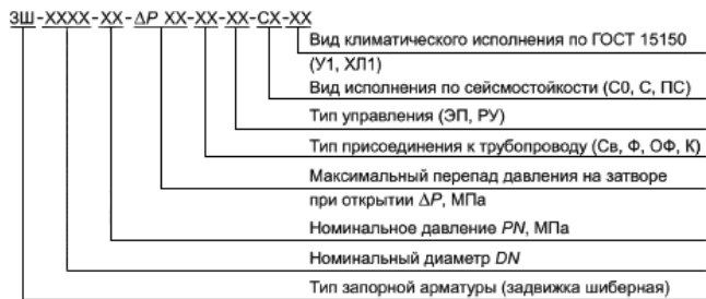
Рисунок 1 - Схема условного обозначения задвижек
